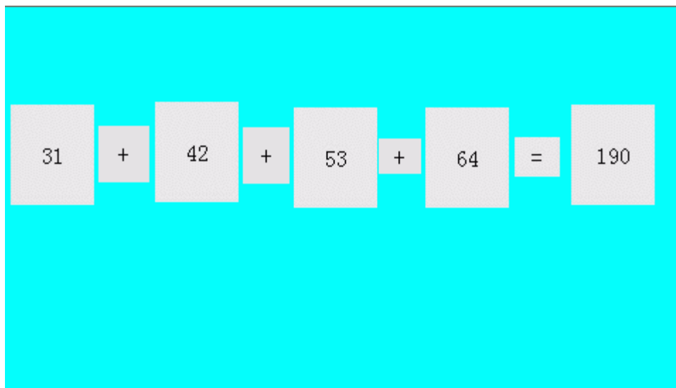
Рисунок 5-21 (Результат вычисления)
