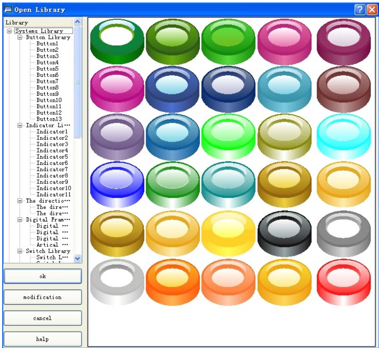
Рисунок 4-43 Список библиотек
