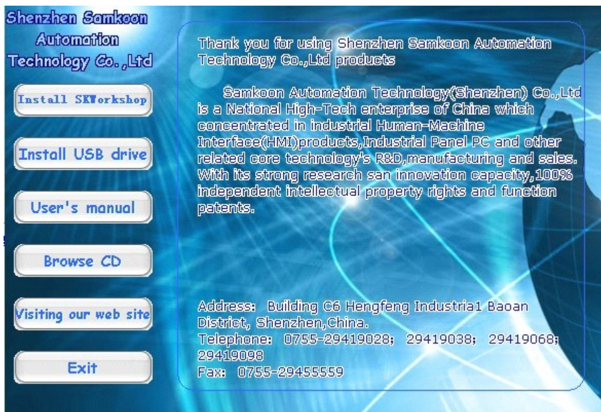
Рисунок 2-2: Автозапуск
