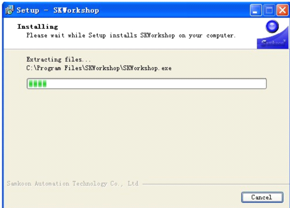
Рисунок 2-10: Окно установки
