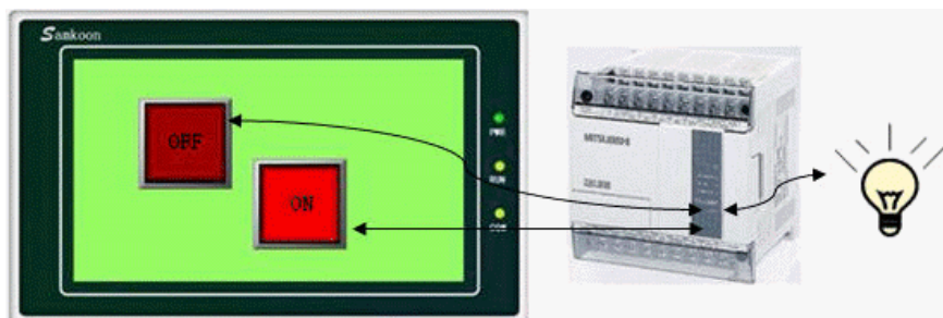
Рисунок 4-83
