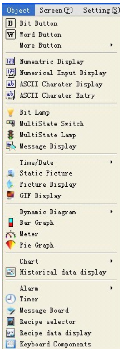
Рисунок 2-32 Меню "Object"
