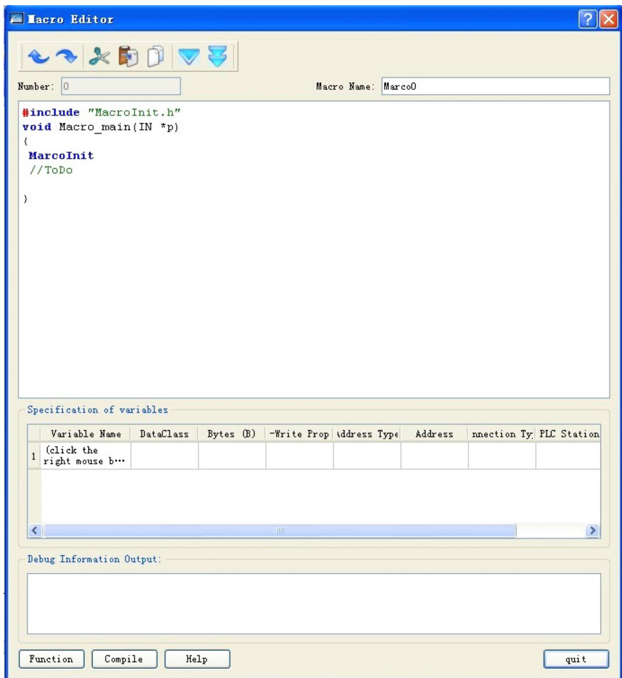
Рисунок 5-4 (компилятор макросов)
