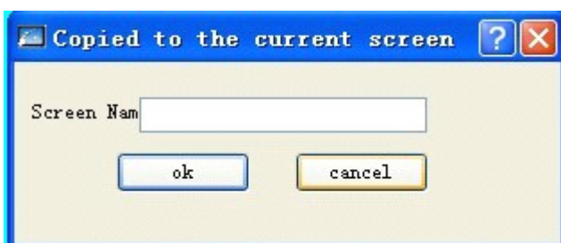
Рисунок 4-5: Копирование экрана
