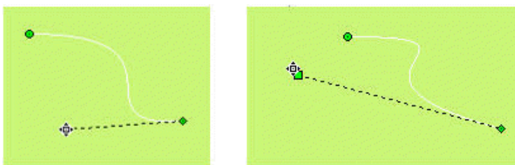
Рисунок 4-27 Рисование кривой/дуги
