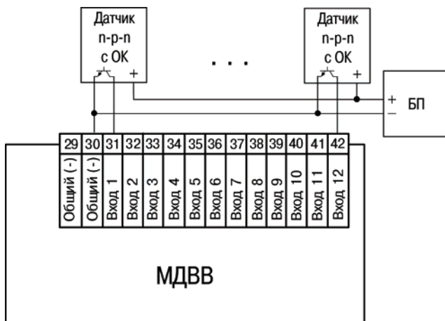
Рис. Б.7. Схема подключения дискретных датчиков n-p-n с ОК
