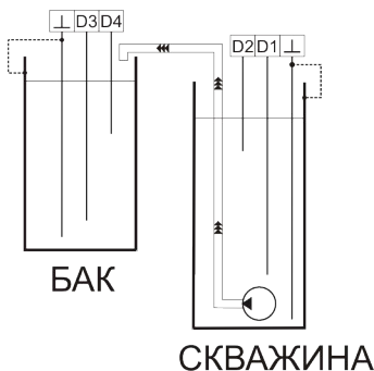
Рис. 5.3 Алгоритм 2: схема подключения
