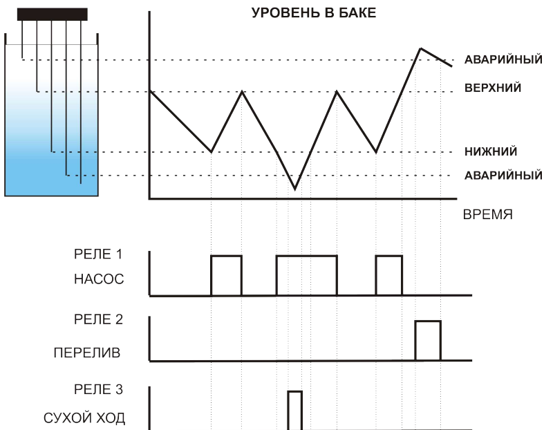
Рис. 5.8 Диаграмма работы алгоритма 4 на заполнение емкости
