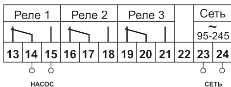
Рис. 5.3 Алгоритм 2: схема подключения
