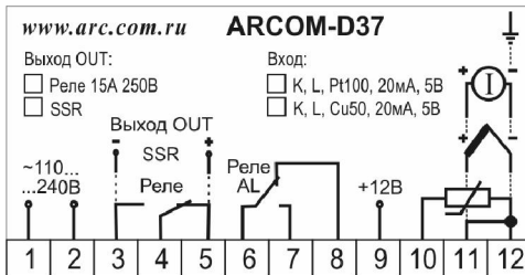
Рис. 2. Схема подключения прибора
